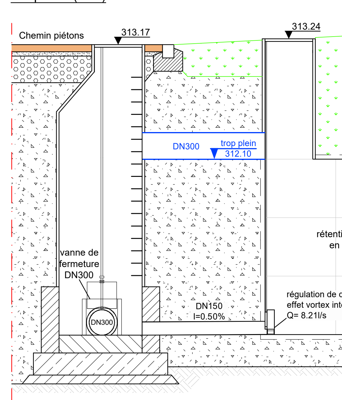
Coupe 3-3 (1:25)
