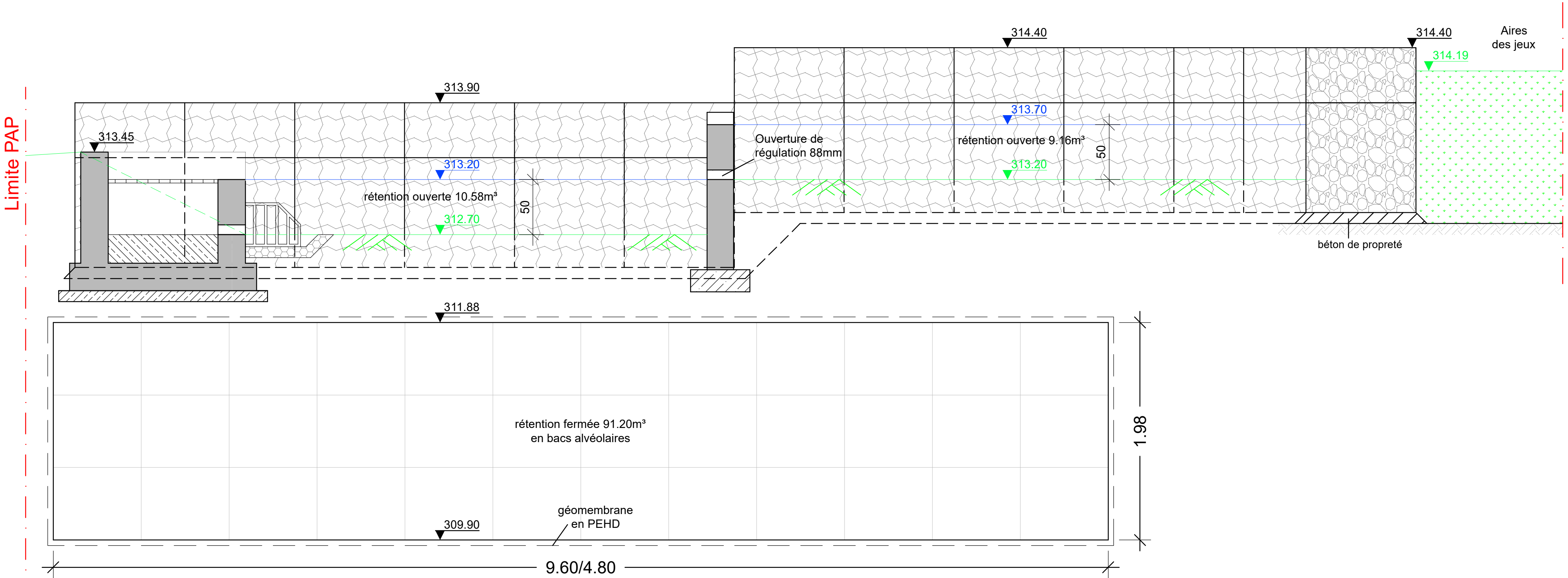
Coupe 1-1 (1:25)
