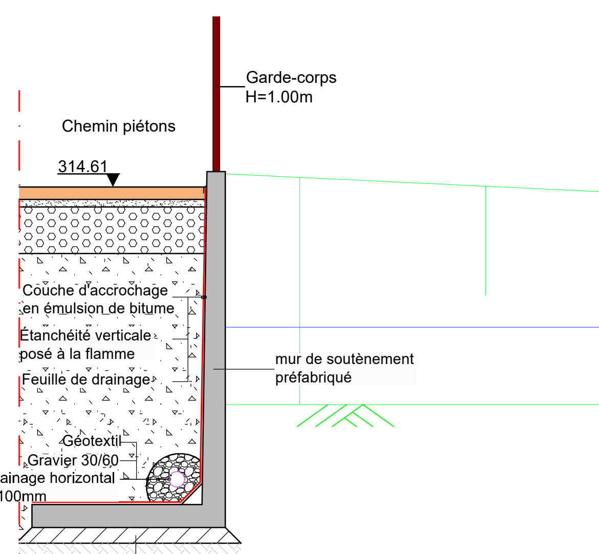
Coupe 3-3 (1:25)
