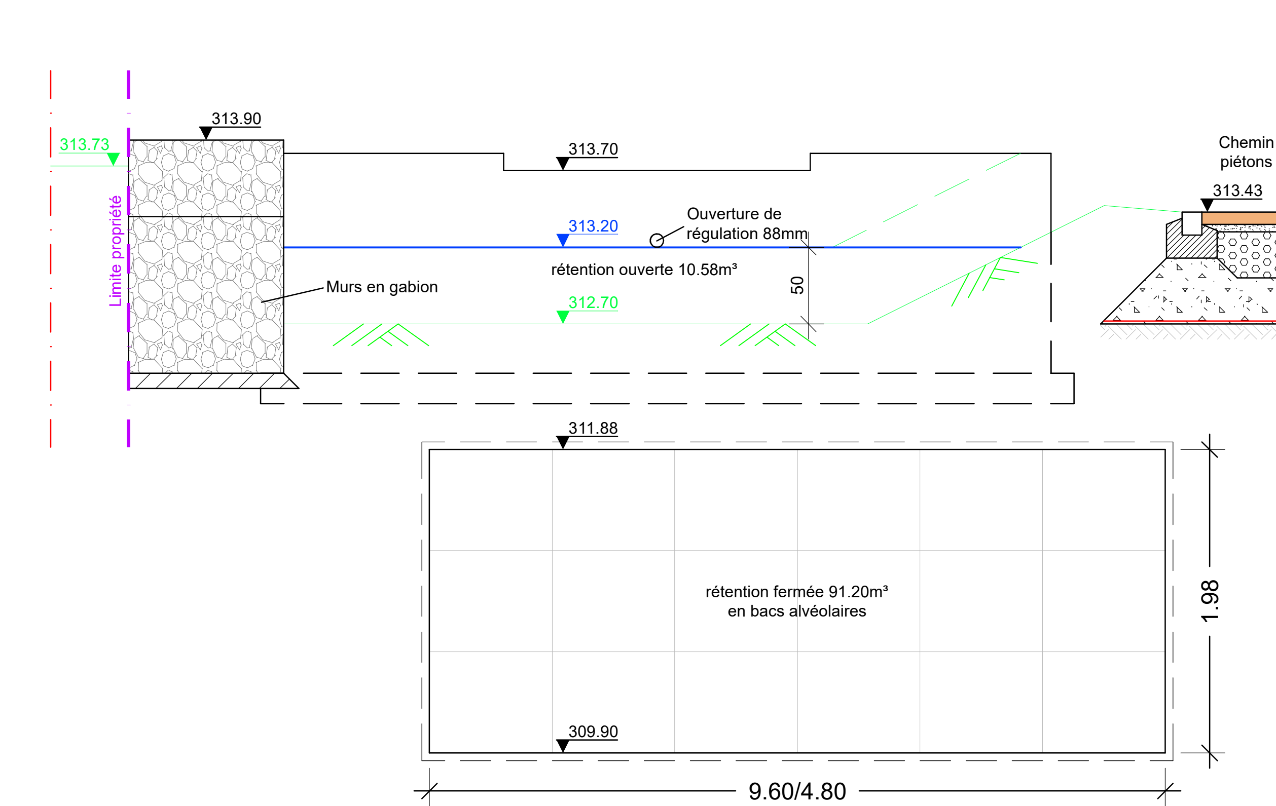
Coupe 2-2 (1:25)
