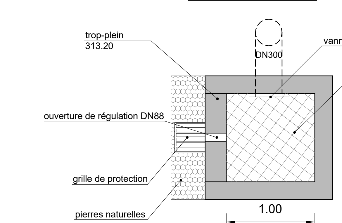
Coupe détail ouvrage rétention ouverte (1:25)
