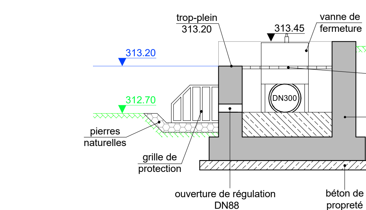
Coupe 4-4 (1:25)
