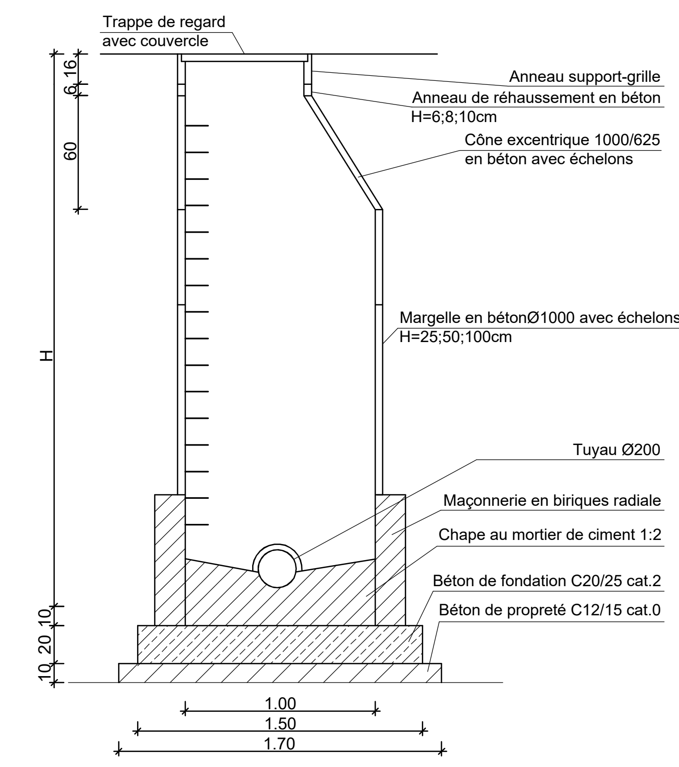
Détail regard (1:20)
